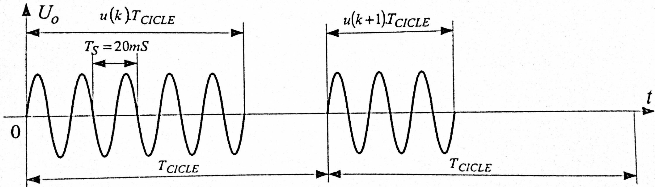
Фиг.7.1. Принцип на циклично регулиране.
