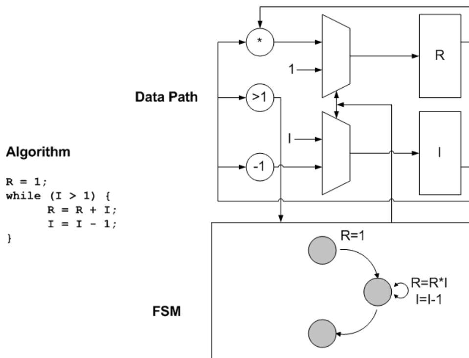
Фиг. 3.9. Хардуерно разпределяне с един множител, един суматор и един компаратор
