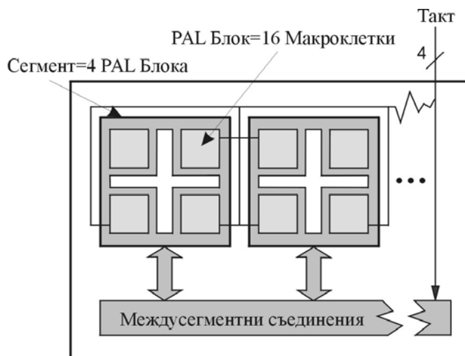
Фиг. 5.9. Архитектура на фамилията MACH5
