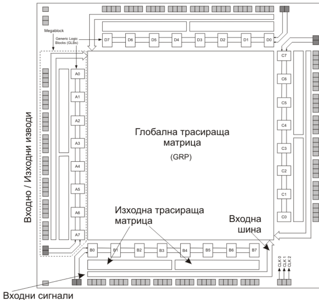
Фиг. 5.11. Архитектура на фамилиите pLSI и ispLSI
