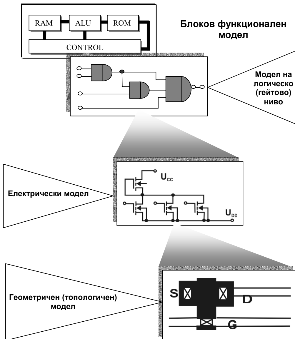
Фиг. 1.4. Системна йерархия на модела
