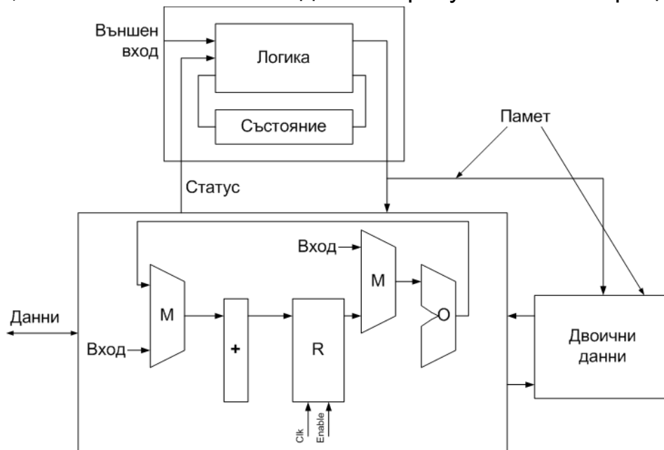
Фиг. 3.7. Структура на схемата създадена от Behavioral Compiler по време на синтеза
