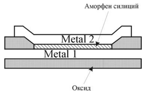
Фиг. 5.33. Antifuse разрез
