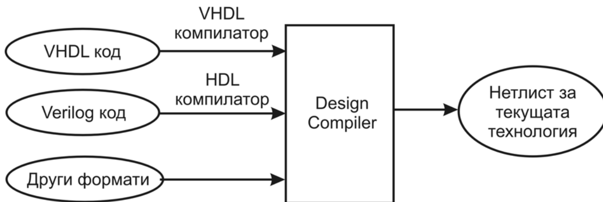
Фиг. 3.1. Design Compiler
