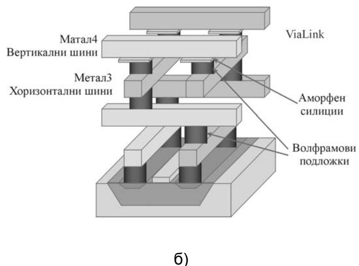
Фиг. 5.34. а) Логически блок на ASIC1 и pASIC2 б) Топология на трасиращите ресурси вете имат и по-нисък паразитен капацитет, както от "PLICE antifuse" ключовете, така и от SRAM и EEPROM технологията.
