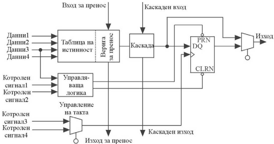
Фиг. 5.27. Организация на логическия елемент
