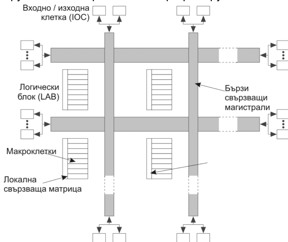
Фиг. 5.5. Базисна архитектура на фамилията MAX9000
