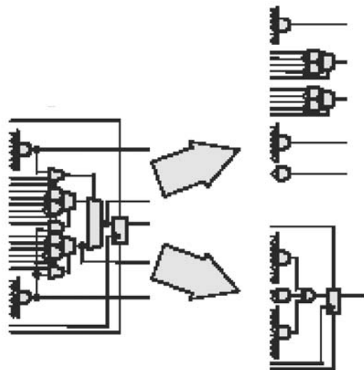
Фиг. 5.35. Логически блок на pASIC3
