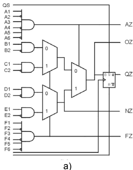
Фиг. 5.34. а) Логически блок на ASIC1 и pASIC2 б) Топология на трасиращите ресурси вете имат и по-нисък паразитен капацитет, както от "PLICE antifuse" ключовете, така и от SRAM и EEPROM технологията.
