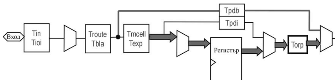
Фиг. 5.19. Времеви модел на CPLD структурата на фирмата Lattice
