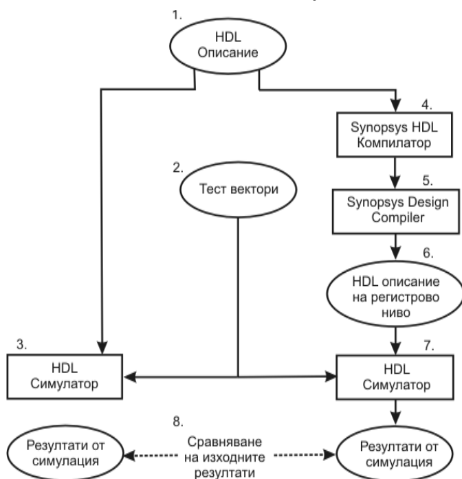
Фиг. 3.4. Типичен пример за употребата на HDL компилатор
