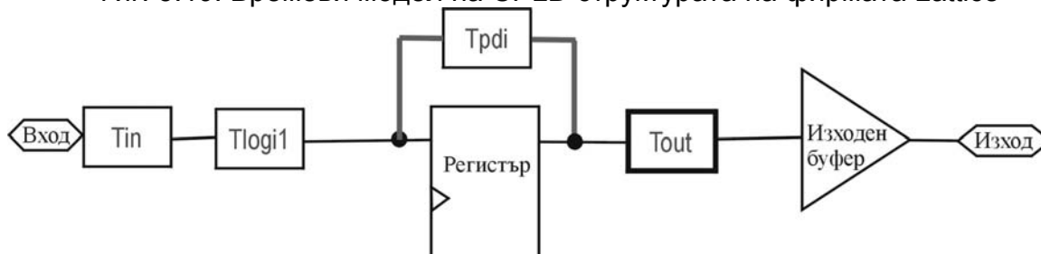
Фиг. 5.20. Времеви модел на CPLD структурата на фирмата Xilinx
