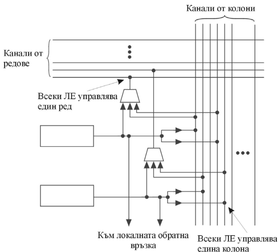
Фиг. 5.26. Организация на логическия блок (ЛБ)
