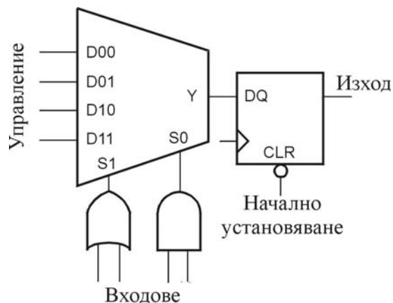
Фиг. 5.30. Структура на логическия блок
