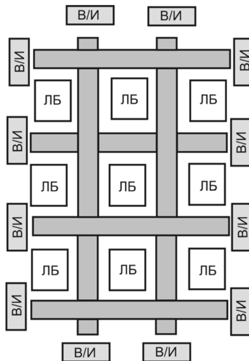
Фиг. 5.32. Архитектура на фамилията pASIC
