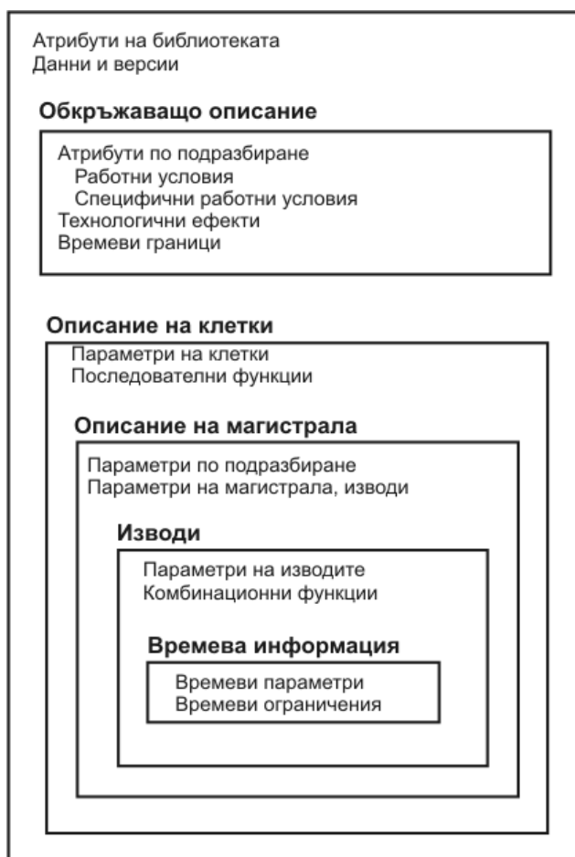
Фиг. 3.12. Структура на технологична библиотека
